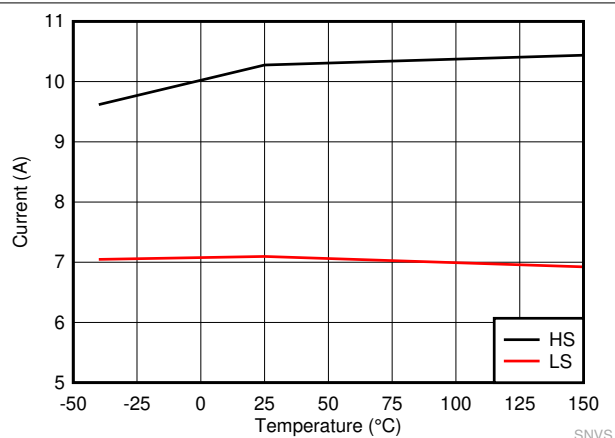
图 6-4. LMQ61460-Q1 高侧和低侧电流限制
