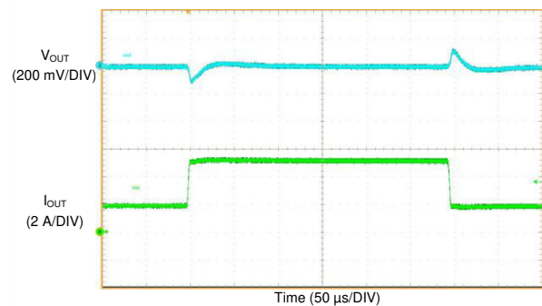
图 8-38. LMQ61460-Q1 负载瞬态
