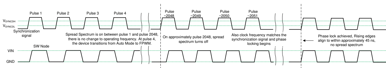
图 7-5. 同步过程
