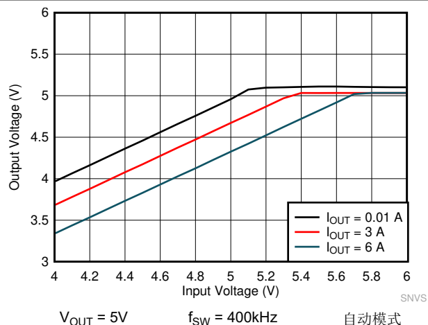
图 8-23. LMQ61460-Q1 压降曲线
