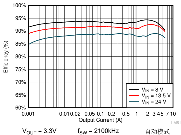
图 8-7. LMQ61460-Q1 效率
