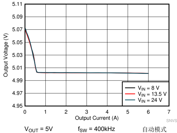
图 8-17. LMQ61460-Q1 负载和线性调整率
