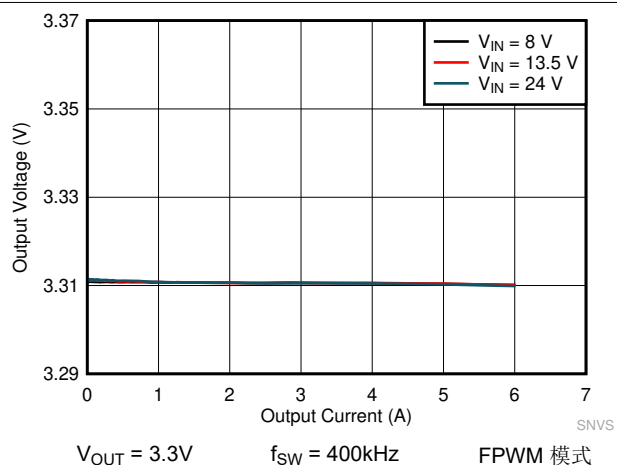
图 8-14. LMQ61460-Q1 负载和线性调整率
