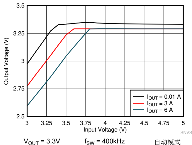
图 8-21. LMQ61460-Q1 压降曲线
