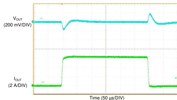
图 8-43. LMQ61460-Q1 负载瞬态
