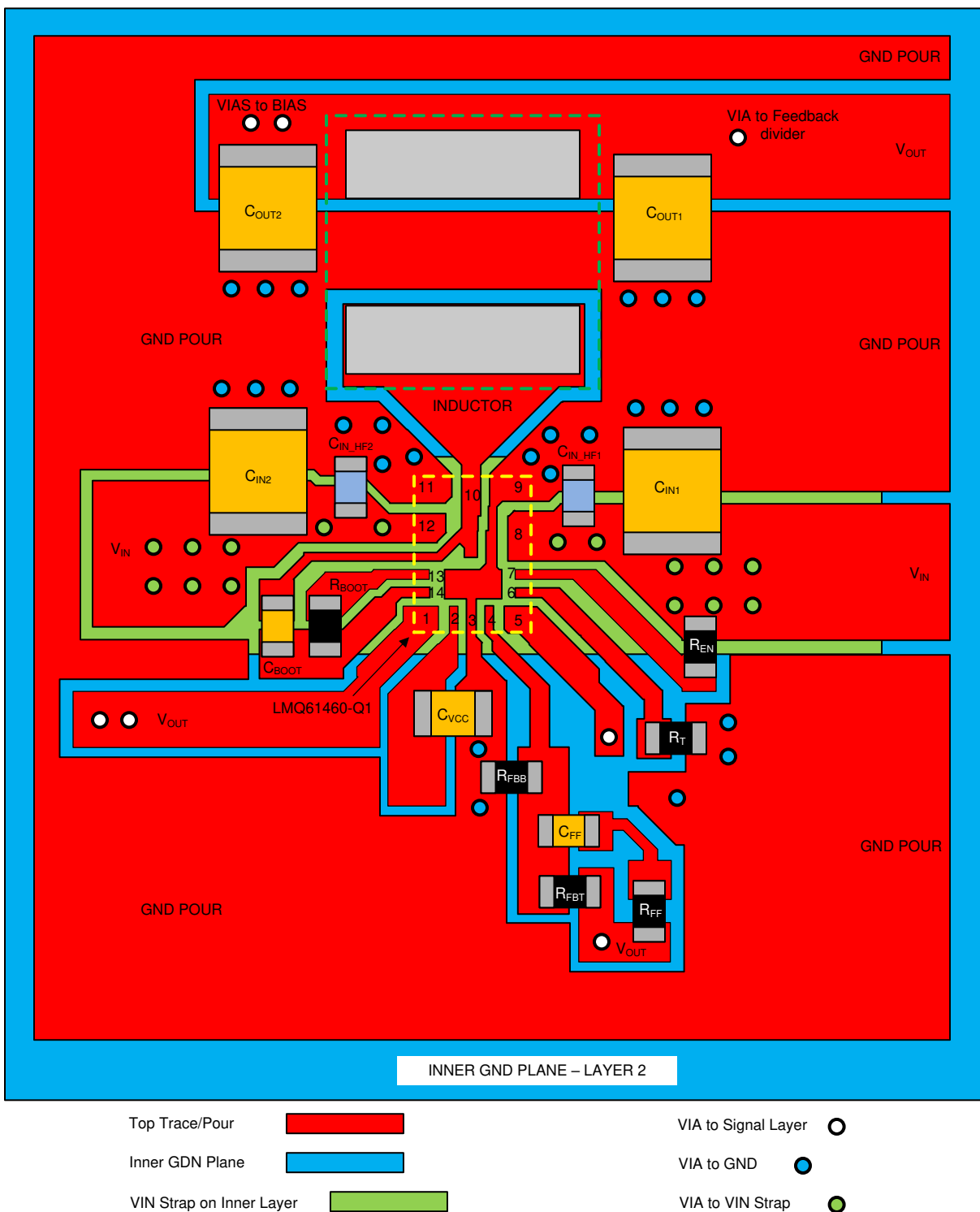
图 8-63. 布局示例
