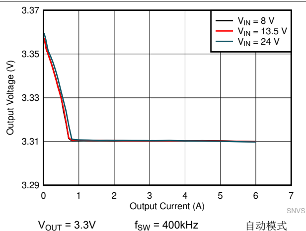
图 8-13. LMQ61460-Q1 负载和线性调整率
