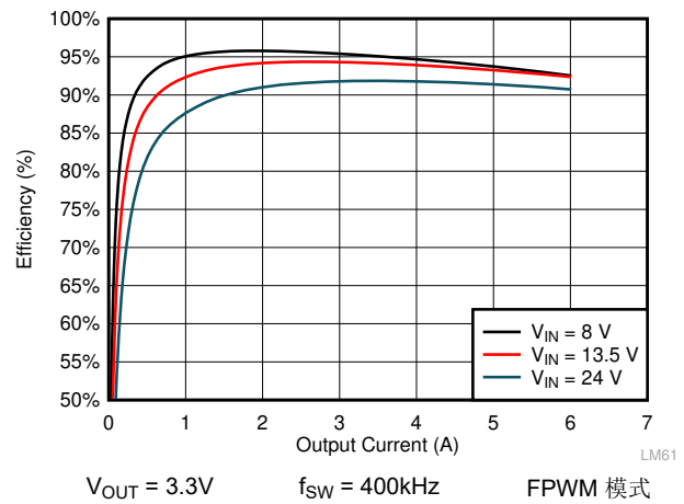
图 8-6. LMQ61460-Q1 效率
