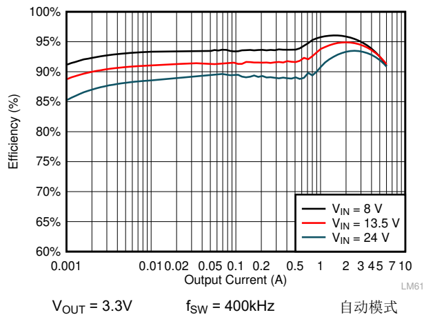
图 8-5. LMQ61460-Q1 效率
