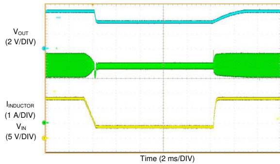
图 8-35. LMQ61460-Q1 短路恢复
