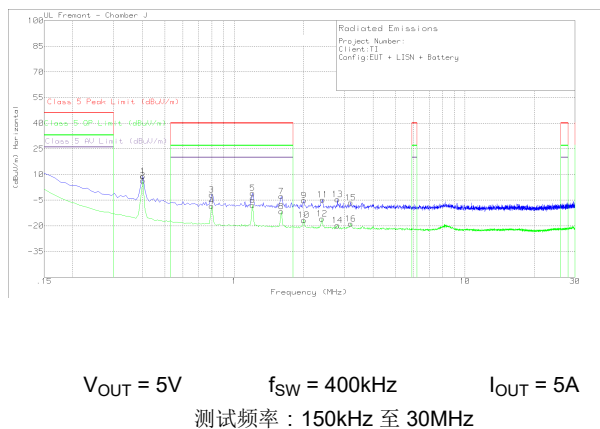
图 8-48. 辐射 EMI 杆状与 CISPR25 限值
