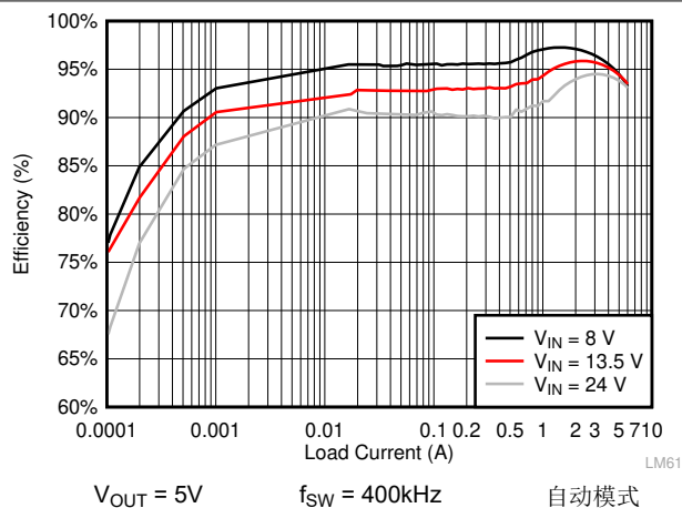
图 8-9. LMQ61460-Q1 效率
