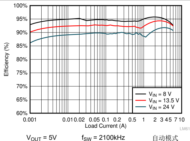
图 8-11. LMQ61460-Q1 效率
