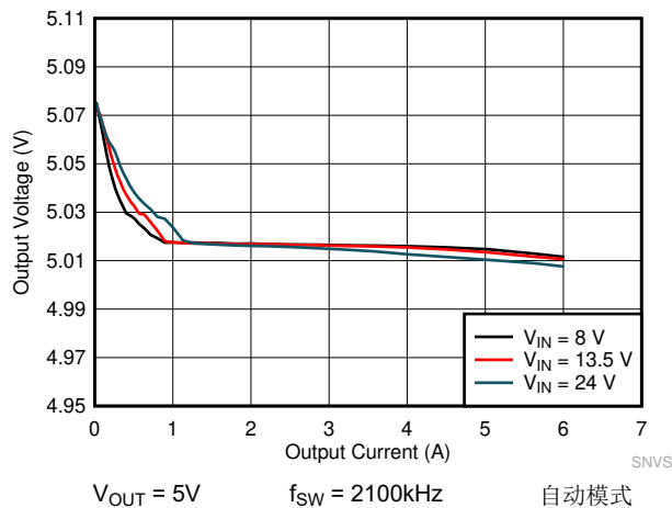
图 8-19. LMQ61460-Q1 负载和线性调整率
