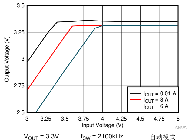
图 8-22. LMQ61460-Q1 压降曲线
