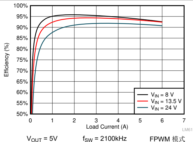
图 8-12. LMQ61460-Q1 效率
