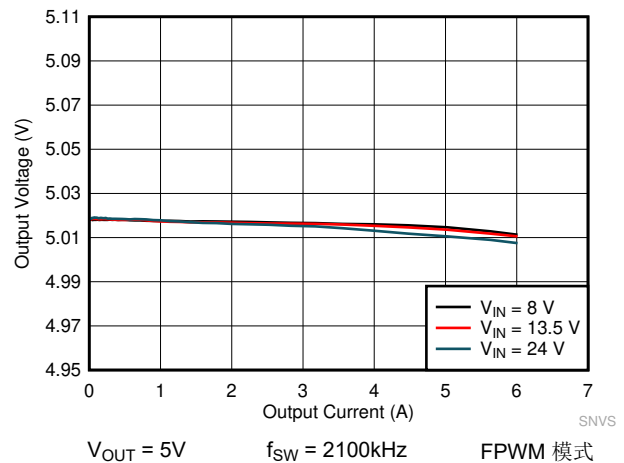
图 8-20. LMQ61460-Q1 负载和线性调整率
