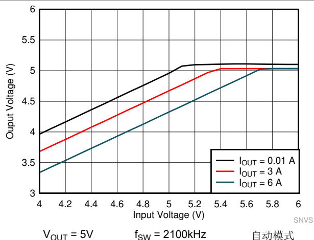
图 8-24. LMQ61460-Q1 压降曲线
