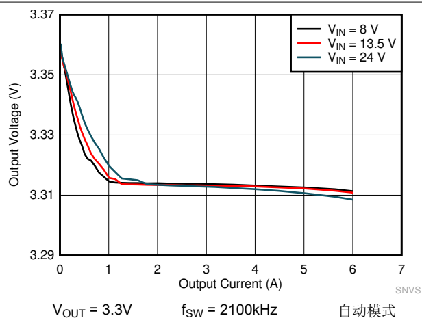
图 8-15. LMQ61460-Q1 负载和线性调整率
