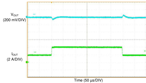
图 8-41. LMQ61460-Q1 负载瞬态
