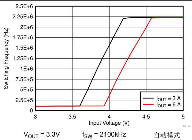
图 8-26. LMQ61460-Q1 压降曲线
