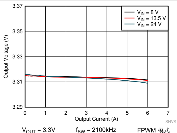
图 8-16. LMQ61460-Q1 负载和线性调整率
