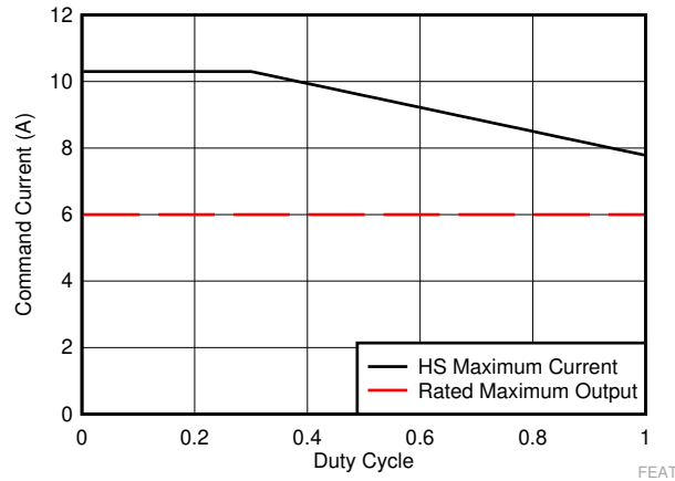
图 7-12. 允许流经 HS FET 的最大电流 - LMQ61460-Q1 占空比的函数
