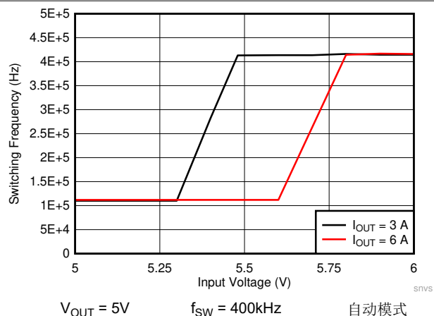
图 8-27. LMQ61460-Q1 压降曲线
