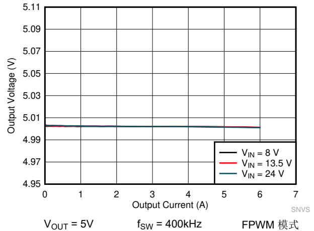
图 8-18. LMQ61460-Q1 负载和线性调整率
