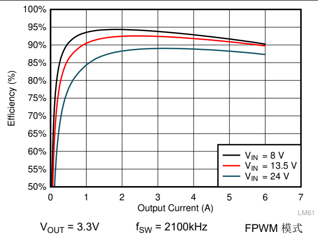
图 8-8. LMQ61460-Q1 效率
