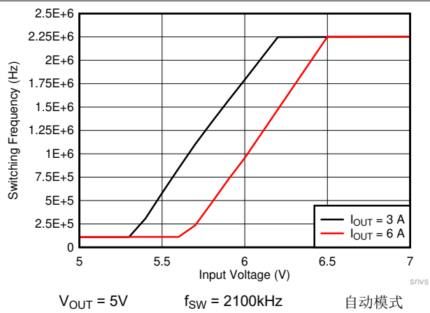
图 8-28. LMQ61460-Q1 压降曲线
