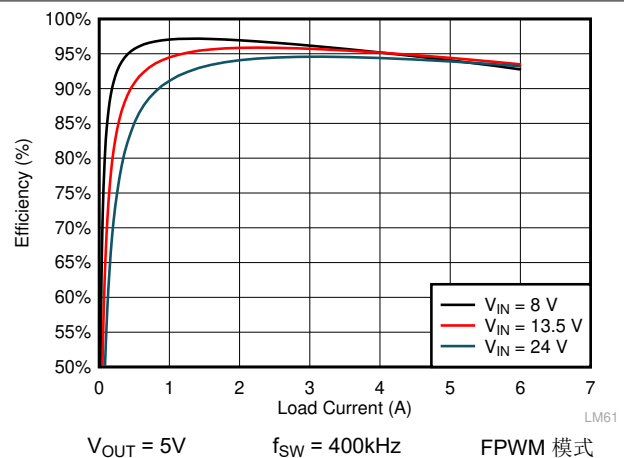
图 8-10. LMQ61460-Q1 效率
