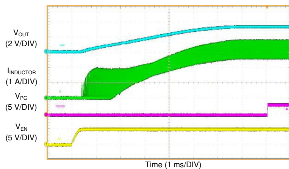
图 8-31. 在 50mA 负载下启动 LMQ61460-Q1
